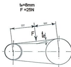
Rys.26 Prawidłowe parametry naciągu pasów
