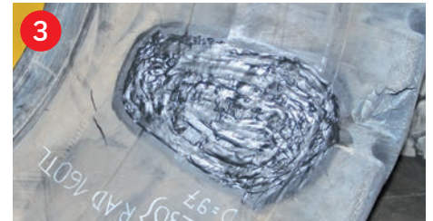
3 Schaden verfüllen und vulkanisieren Fill injury und vulcanize
