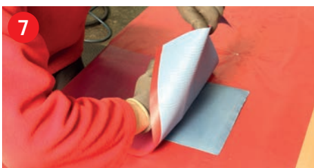
7 Pflaster mit Cement streichen und doublieren Coat patch with cement and laminate
