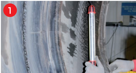
1 Fremdkörper entfernen / Bereich reinigen / Schaden markieren Remove foreign object / Clean area / Mark injury
